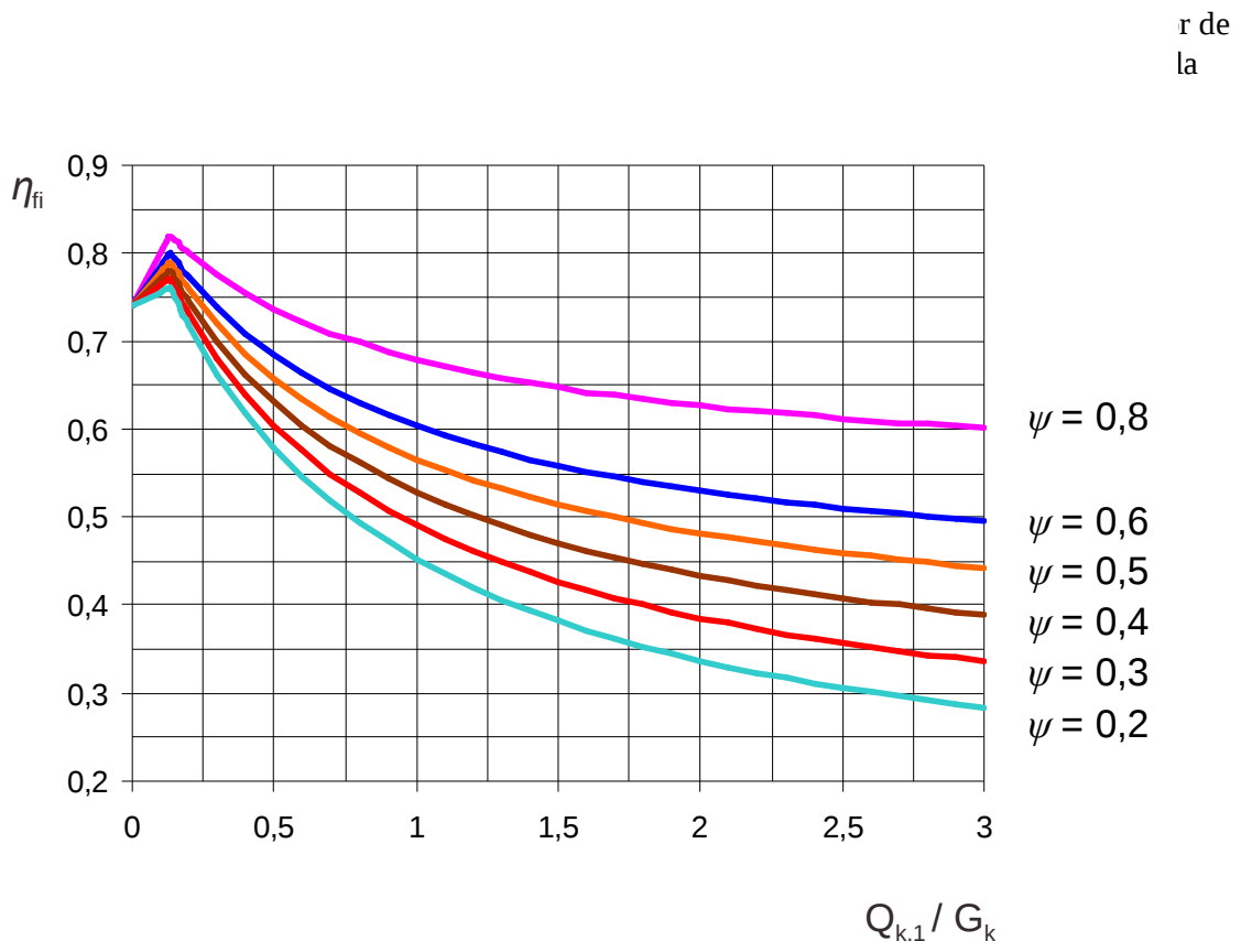
Figur 1-FI: Exempel på värden för reduktionskoefficienten \eta_{fi} som funktion av lastförhållandet Q_{k1}/G_k för de värden, som finns i de nationella bilagorna till standarderna EN 1990 och EN 1991-1-2.
